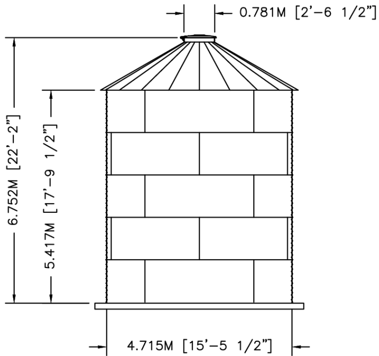
ELEVATION
